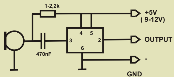
Montaż dla mikrofonu elektretowego
