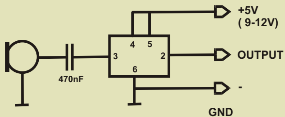
Montaż dla mikrofonu dynamicznego
